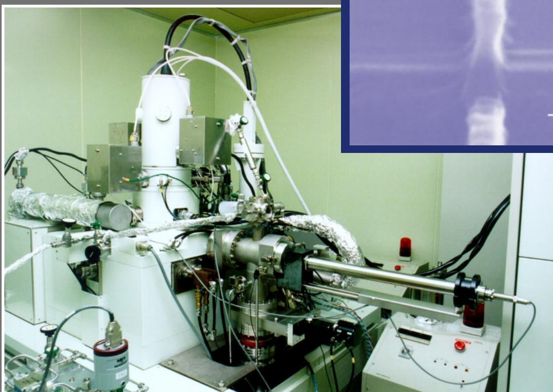
電子ビーム露光装置
