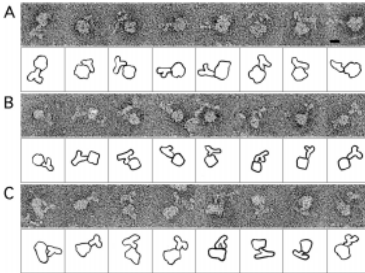
図5 生電子顕微鏡写真からの抗体とNaチャンネルの結合像 抗体はNaチャンネルのアミノ酸配列の一部に対してつくられた。抗体とNaチャンネルが結合していることが判る。Y字型のものが抗体であり、それが結合している円筒状のものがNaチャンネルである。右上のスケールバーは10nmを表わす。 A : Naチャンネルをほぼ上方から見た図、B : Naチャンネルを下方より見た図、C : Naチャンネルを側方より見た図
