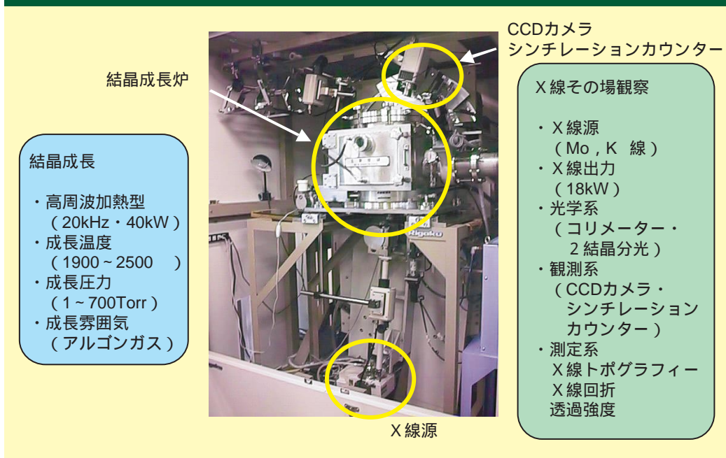
図3 X線トポグラフィー結晶成長その場観察装置
