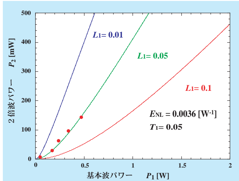
図2 2倍波パワーと基本波入力パワーの関係
