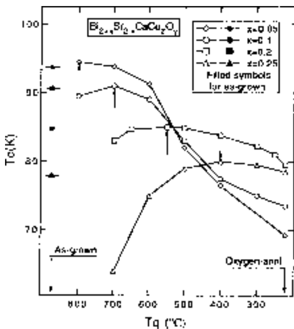
図 11 \text{Bi}_{2-x}\text{Sr}_{2-x}\text{CaCu}_2\text{O}_y の x (Bi/Sr 比) を変えたいくつかの試料について、更にその熱処理温度 ( T_q ) によって酸素濃度 ( y ) を変えたときの超電導転移温度の変化。矢印はそれぞれの Bi/Sr 比のときの最高転移温度 (最適酸素量) の試料。矢印の右側が過剰酸素 (Overdoped) の試料、左側が欠乏酸素 (Underdoped) の試料であり、酸素濃度が広範囲で制御されている。転移温度 95 K はこの系での初めての最高値である。(Ref.25)
