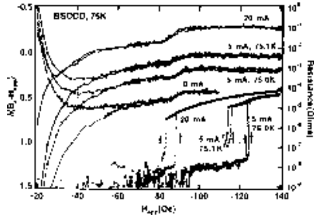
図 12 \text{Bi}_2\text{Sr}_2\text{CaCu}_2\text{O}_y の広い c 面をもつ短冊状の試料面に垂直に磁場 ( H_{tr} ) を加え、磁束格子融解転移近傍での試料中心の局所磁化 (微小ホー ル素子による) と電気抵抗を同時に測定したもの。磁化ステップでみられる転移磁場と電気抵抗のステップでみられる転移磁場の差は、表面障壁などのため試料内での磁束分布と電流分布が一様でないためと考えられる。(Ref.28)
