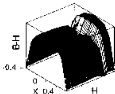
図14 微小ホール素子アレイで測定したOverdope -Bi 2 Sr 2 CaCu 2 O y の磁化曲線。挿入図は板状試料とホール素子との相対関係。磁化は試料中心で高く試料端で低いドーム状になっているが、不可逆磁場(融解転移が重なっている)直下(1400 Oe近傍)では磁束ピン止め効果のため、ピンモデル型(V字型)のプロファイルが少し重なっている。(Ref.31)
