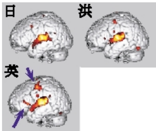
図2 健常人被験者における、日本語、英語、ハンガリー語の聴覚理解時における脳活動の一例
